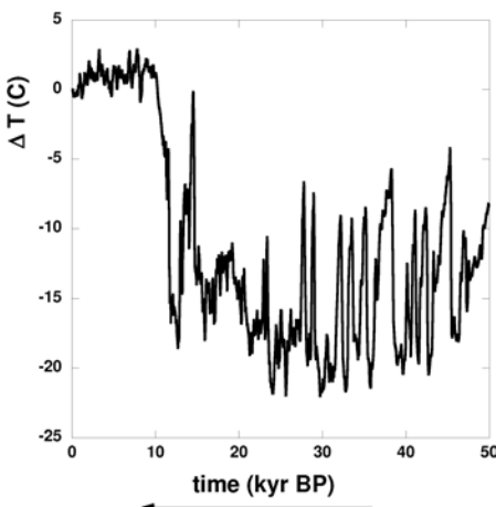
Figuur 1 Temperatuurafwijking t.o.v. het gemiddelde over de laatste 100 jaar op een lokatie in centraal Groenland, zoals gereconstrueerd uit ijskernen (1 kyr = 1000 jaar).
