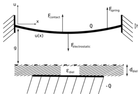
Figuur 1 Schematische doorsnede van een capacitieve RF MEMS schakelaar
