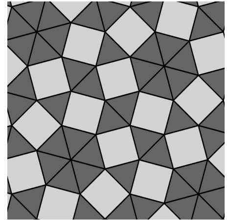
Figuur 2 Voor een vierkant-driehoekbetegeling is een twaalfvoudige rotatiesymmetrie mogelijk (figuur: B. Nienhuis)
