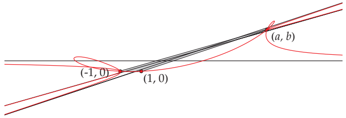
Figuur 4 De zevendegraads kromme \Gamma met basispunten (-1, 0) , (1, 0) en (a, b) en de drie asymptoten voor a = 13 en b = 4 .
