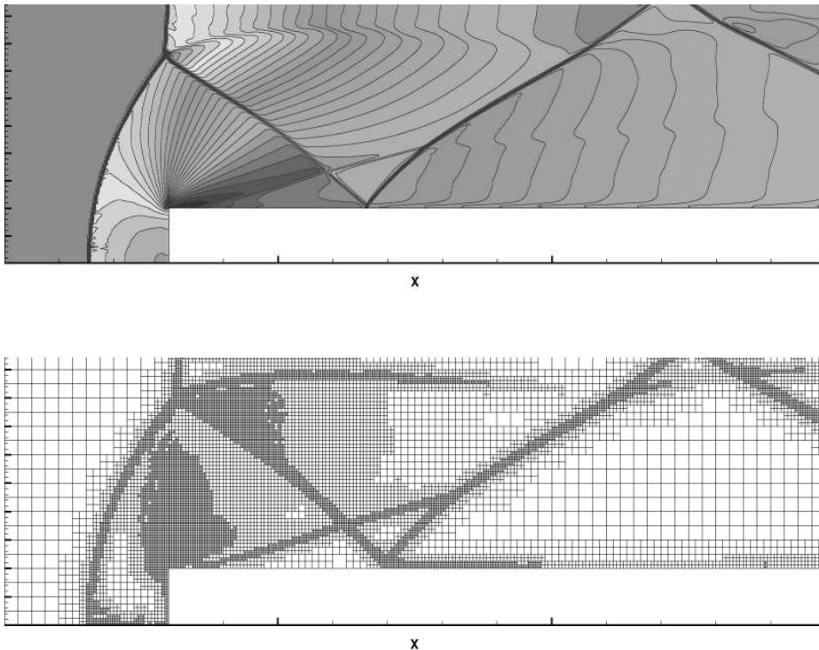
Figuur 11 Rekenresultaat enige tijd na instantaan afsluiten van onderste deel van kanaaltje. Boven : isolijnen van luchtdichtheid. Als het verticale klepje nog openstaat is de luchtdichtheid in het hele kanaaltje constant. Onder : automatisch aan stroming aangepast rooster.
