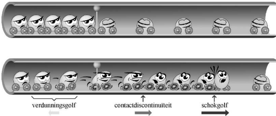
Figuur 7 'Schokbuis'. Boven : rusttoestand met in linker en rechter gedeelte: hoge respectievelijk lage druk en dichtheid. Onder : bewegingstoestand met naar rechts lopende shokgolf en contactdiscontinuïteit en naar links lopende verdunningsgolf.
