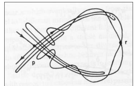
Figuur 1 Een homokliene baan
