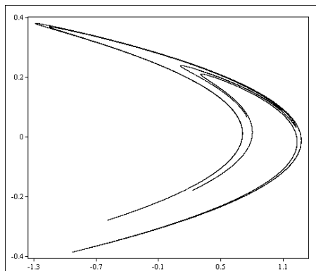
Figuur 2 De vreemde aantrekker van Hénon
